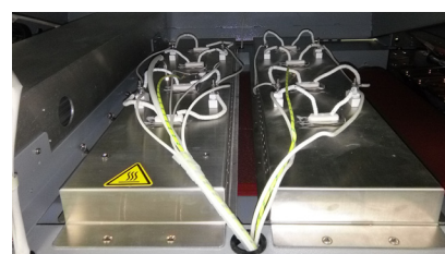
Kit de Doble IR opcional para impresiones por KMBS y Ricoh
